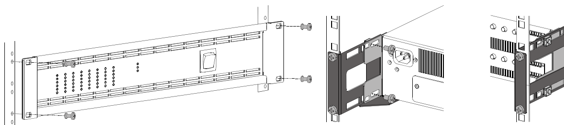
Abbildung 2.1: Befestigung der Endstufe bei Rackeinbau
